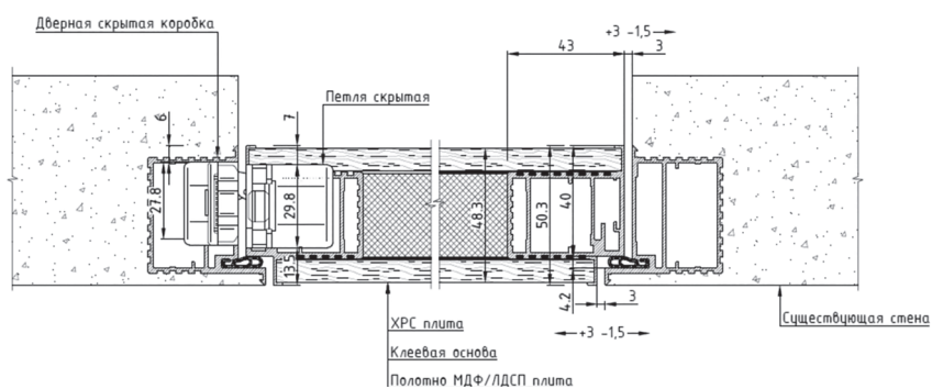
Схема внутреннего открывания (IN)
