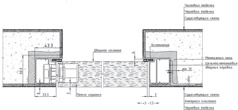
Схема внутреннего открывания (IN)
