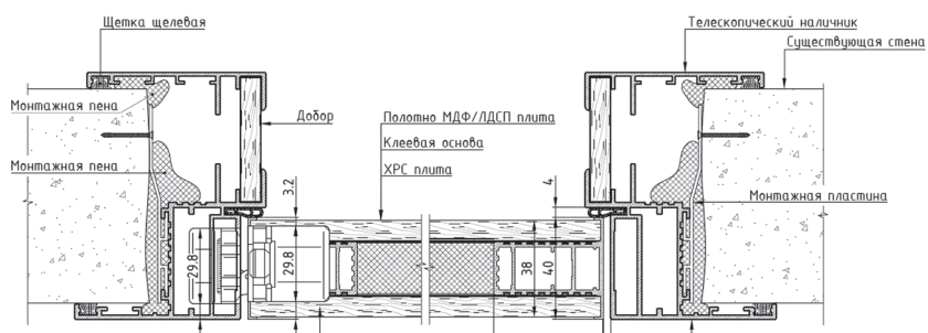
Схема внутреннего открывания (IN)
